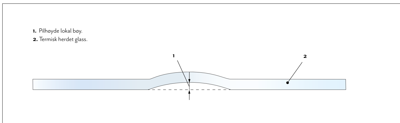
Figur 17: Lokal bøy forårsaket av vertikal herdeprosess.
